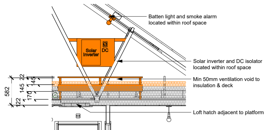
2 Solar Inverter Callout 1 : 50
